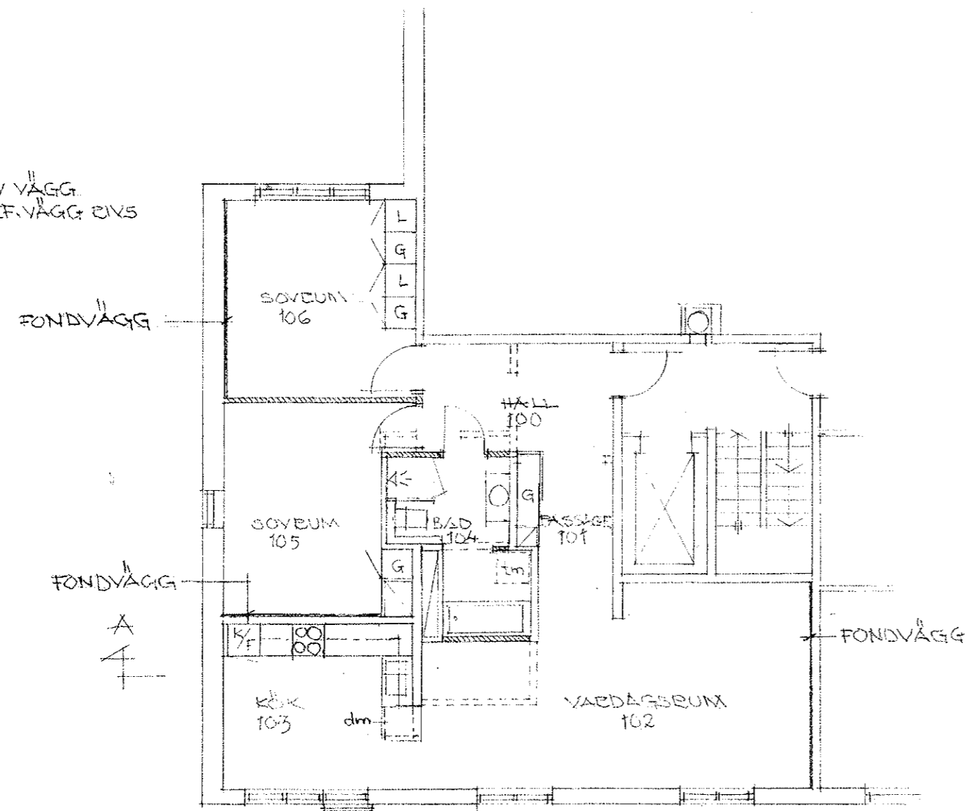
PLAN SK 1:100
