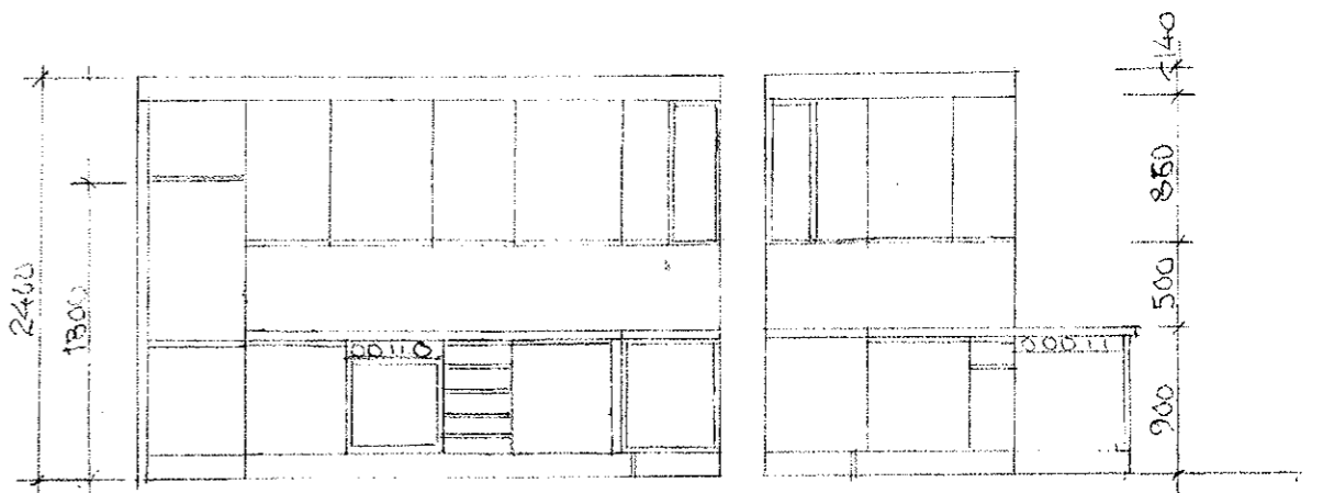
FASAD A KÖKSUPPSTÄLLNING SK 1:50
